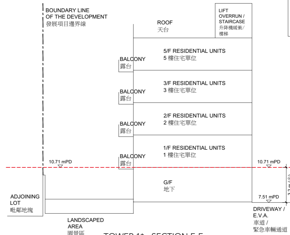
TOWER 1* - SECTION E-E 第1座* - 橫截面圖E-E
