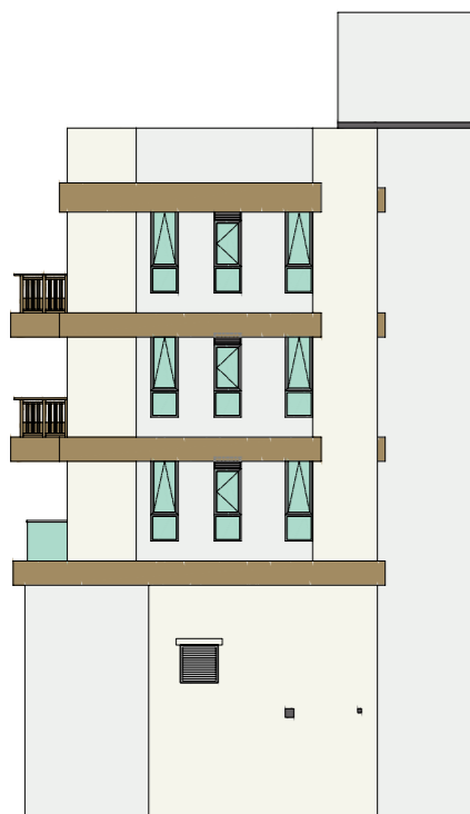
ELEVATION 2 立面圖 2
