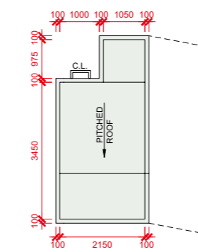
UPPER ROOF PLAN 上層天台平面圖
