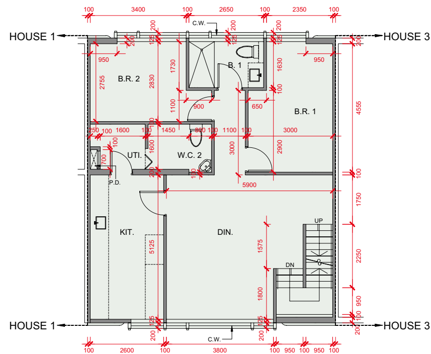
1/F PLAN 1樓平面圖
