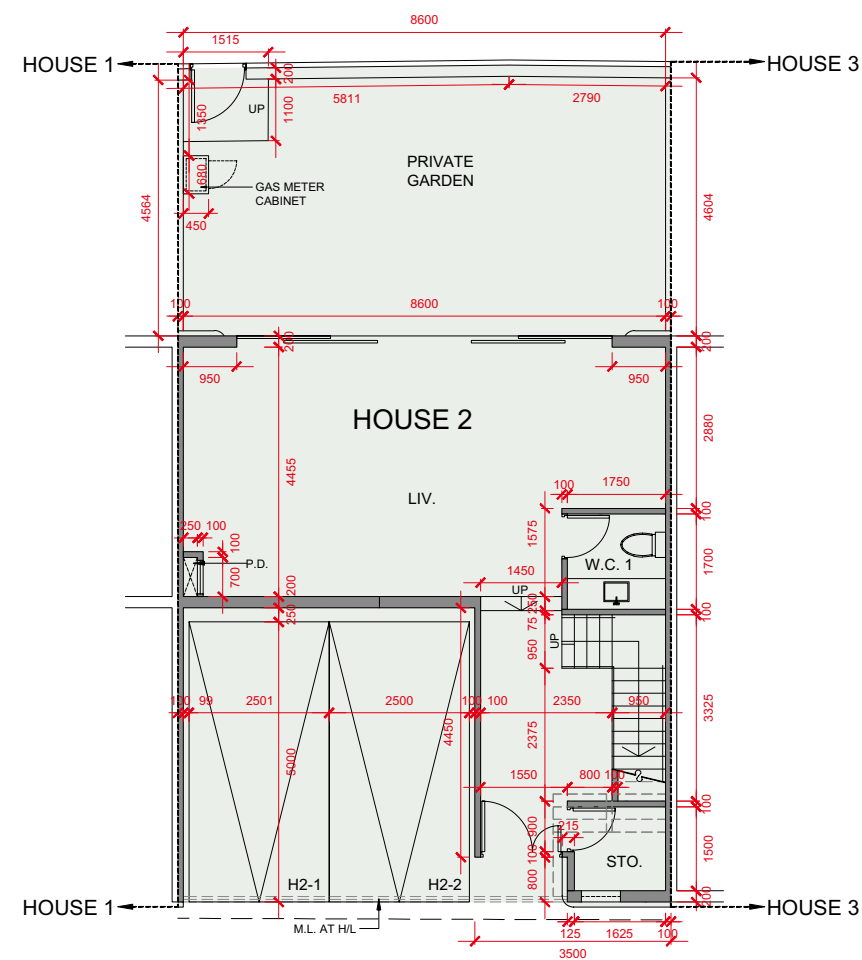
G/F PLAN 地下平面圖
