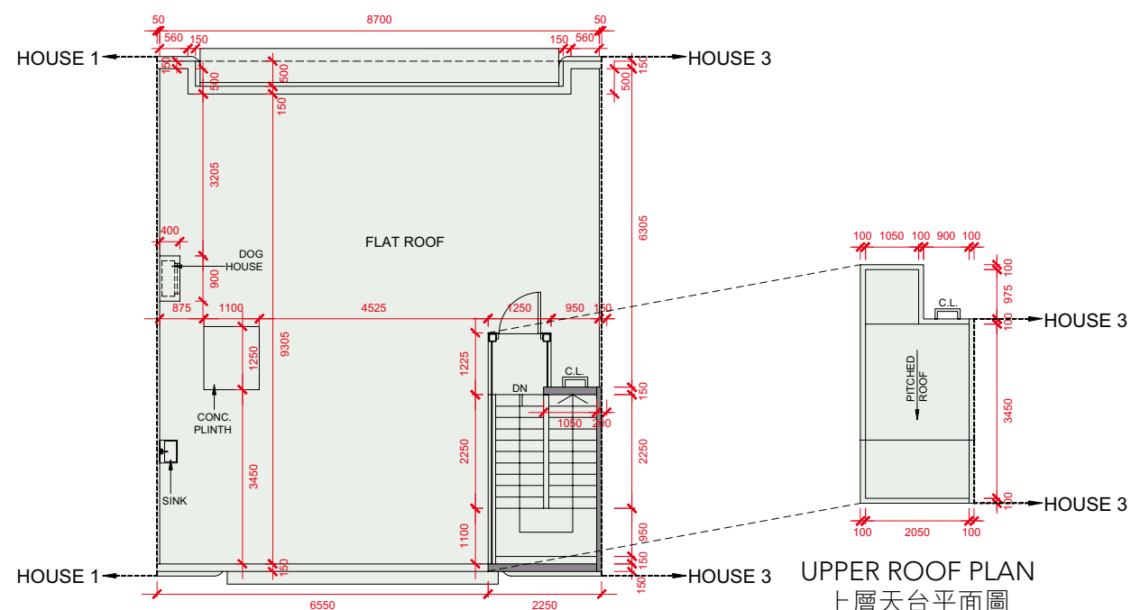
ROOF PLAN 天台平面圖
