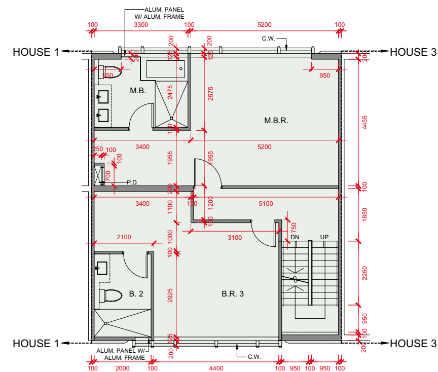
2/F PLAN 2樓平面圖
