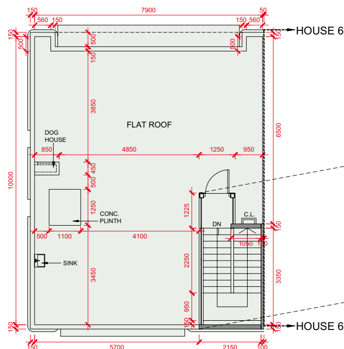
ROOF PLAN 天台平面圖
