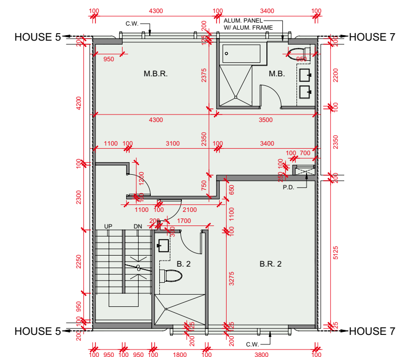
2/F PLAN 2樓平面圖
