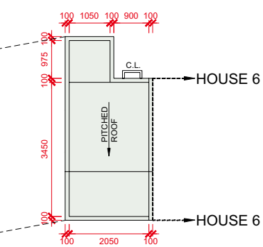
UPPER ROOF PLAN 上層天台平面圖
