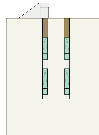
ELEVATION 4 立面圖 4
