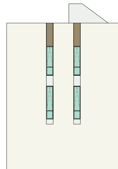
ELEVATION 4 立面圖 4
