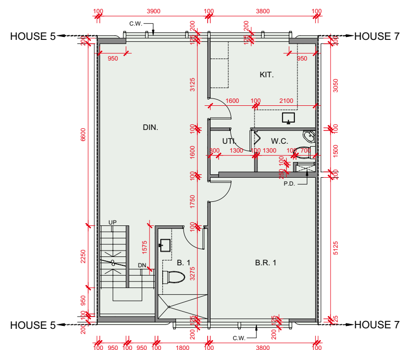
1/F PLAN 1樓平面圖
