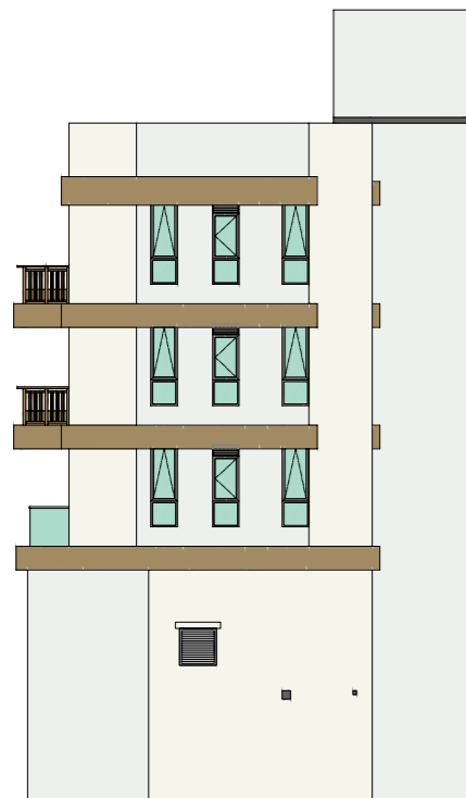
ELEVATION 2 立面圖 2
